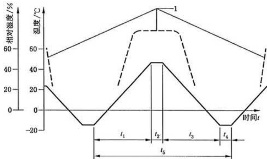
图 7 水气密封耐久性试验温度曲线
