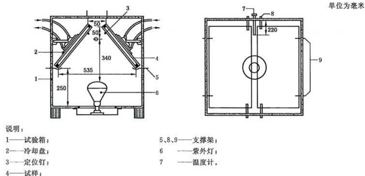
图 5 紫外线试验箱
